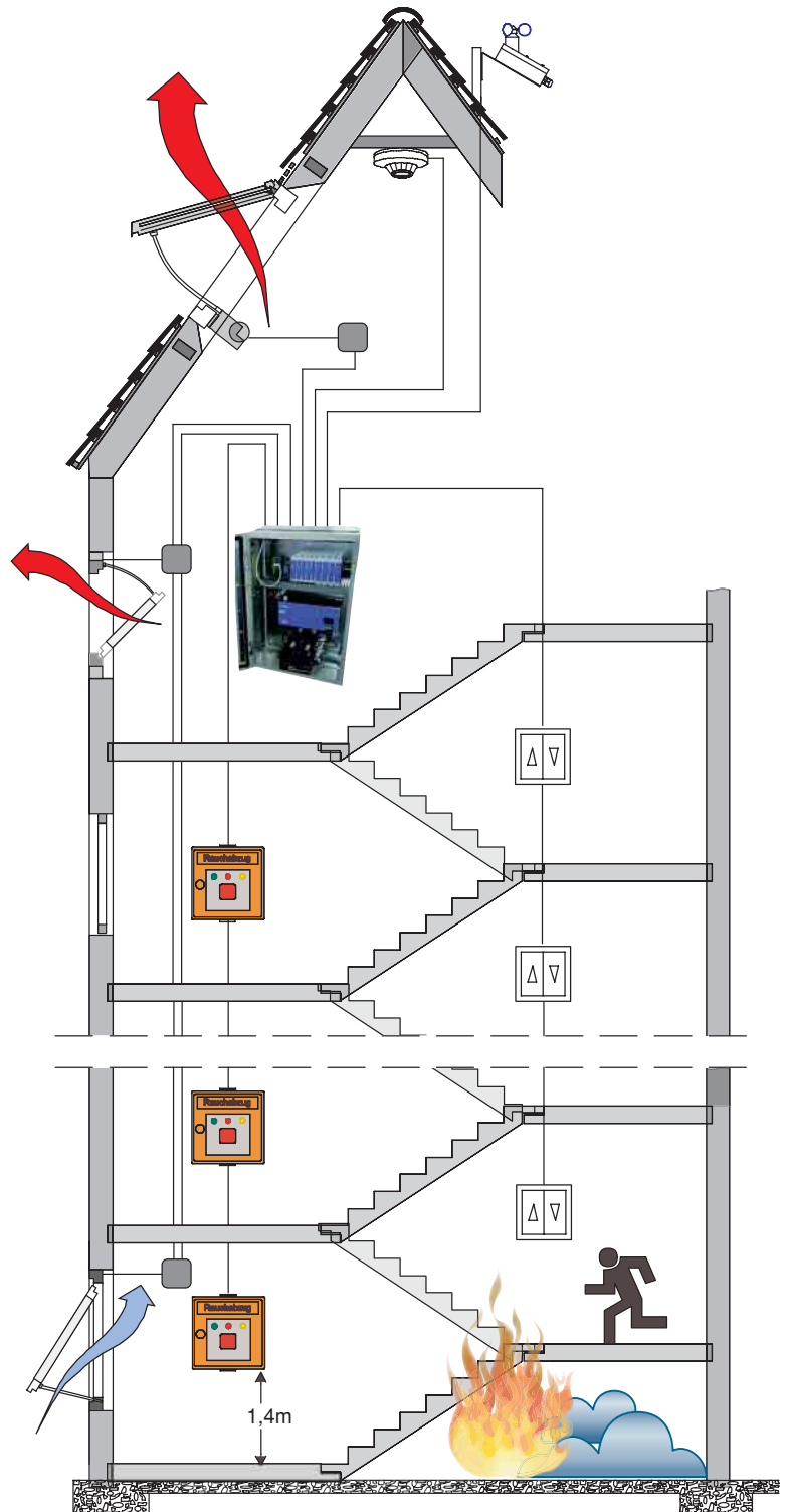
Anwendungsbeispiel Schüco RWA Example of Schüco SHEVS
